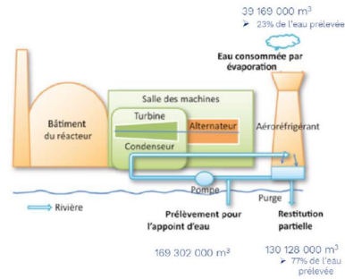
CNPE de Belleville – 2x 1300 MW – circuit dit « fermé » – Loire
