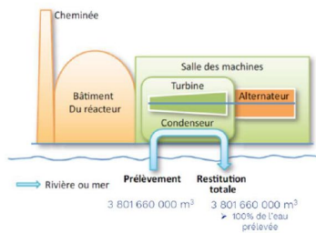
CNPE de Saint-Alban – 2x 1300 MW – circuit ouvert – Rhône
