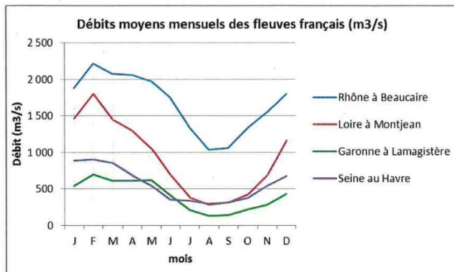
Débits moyens des fleuves français et débit moyen en août (source : Agence de l'eau Rhône-Méditerranée-Corse)
